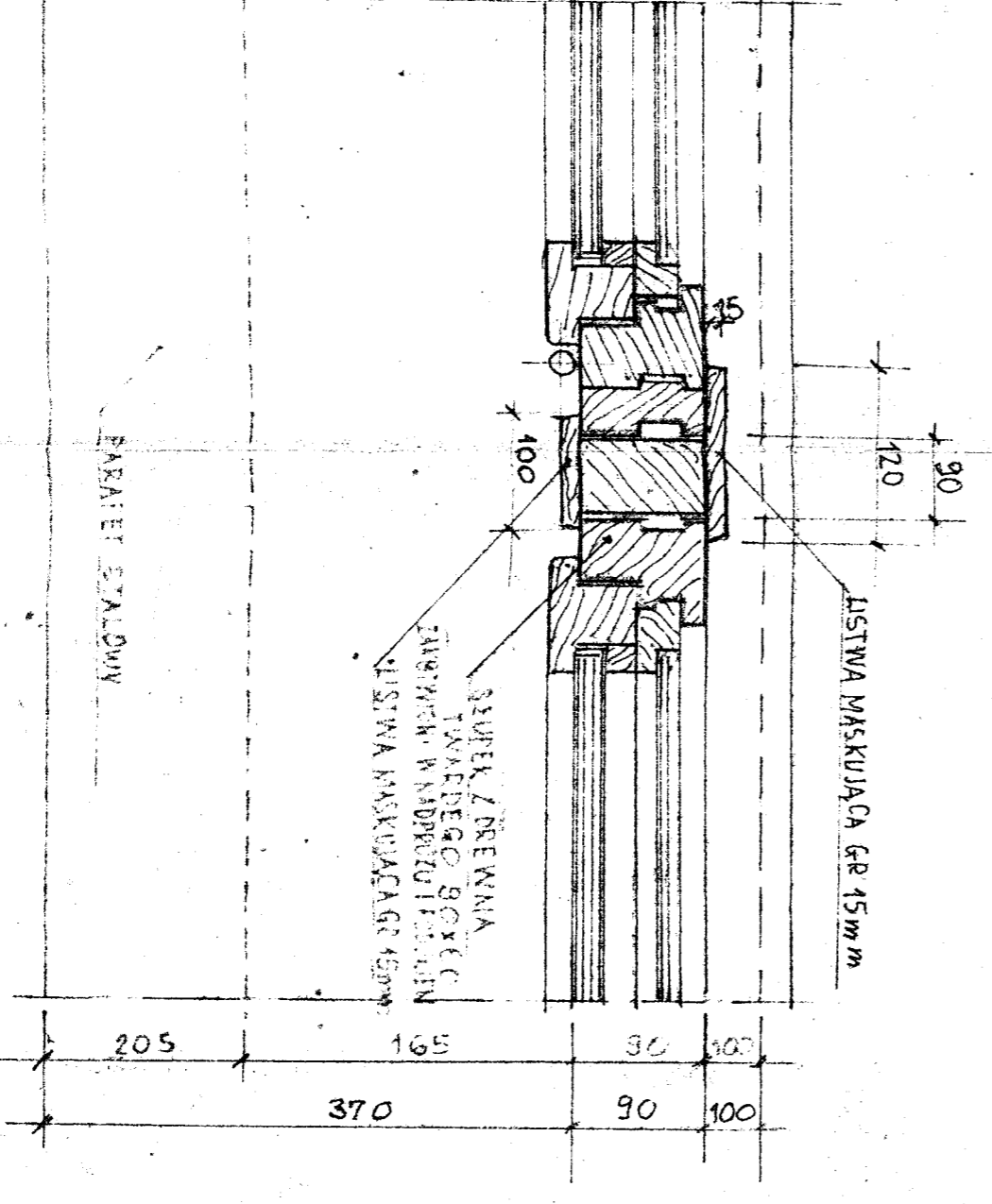
OKNA ZESPOLONE ZE ŚLUPKIEM DREWNIANYM SZER. 60mm SKALA 1:5
